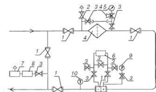
Схема пневматическая функциональная узла учета расхода газа с суживающим устройством:
